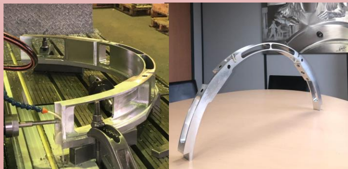
Usinage pièce aluminium
